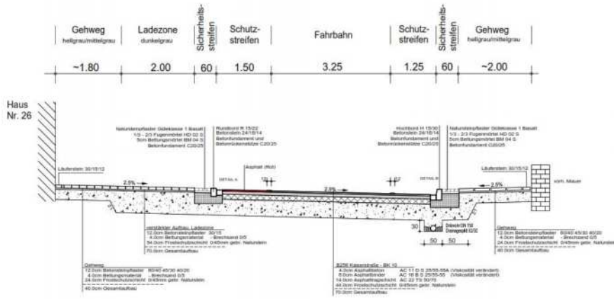
Kaiserstraße Regelquerschnitt 0+085.000
