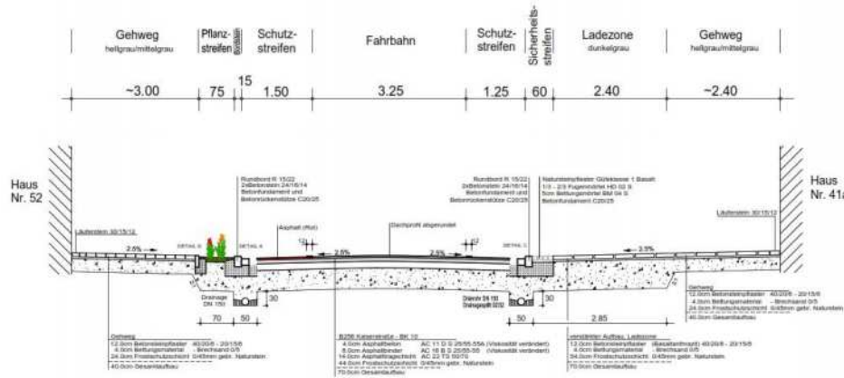
Kaiserstraße Regelquerschnitt 0+410.000
