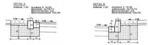
Details der Randeinfassung
